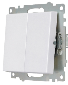
کلید دو پل روشنایی MC2LS00W02
